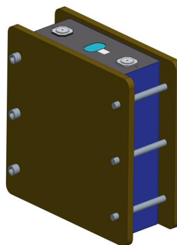
图 4 电池带夹具示意图
