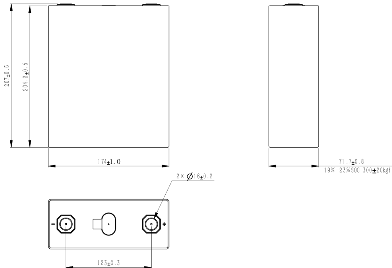
图 8 电池尺寸及外观图
